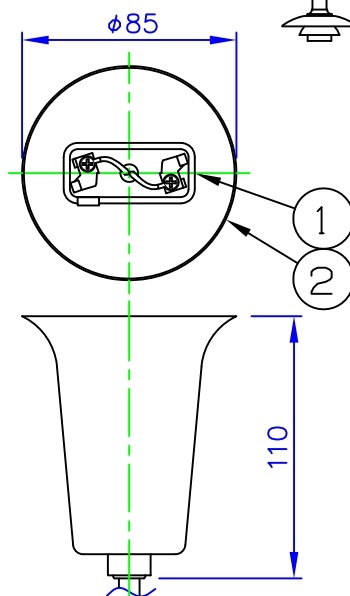
フランジ寸法図
