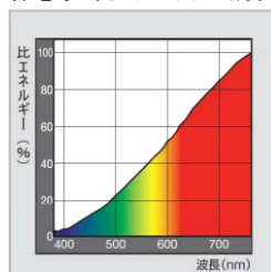
白熱電球
